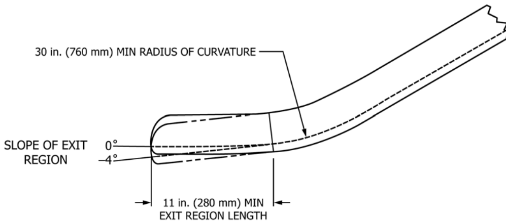
FIG. A1.22 Slide Exit Requirements Sections 8.5.11.2, 8.5.11.3, 8.5.11.4
